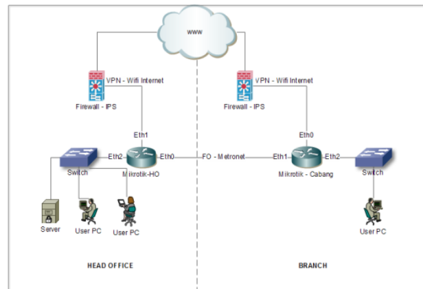
Gambar 2. Skema Jaringan Metronet Fiber Optik dan VPN
