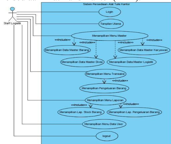
Gambar 1. Use Case Diagram Sistem Informasi Persediaan ATK
