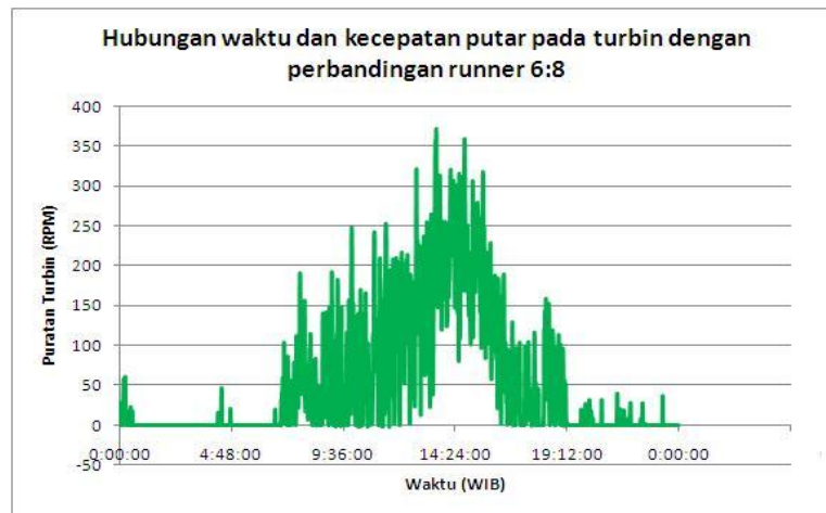
Gambar 3. Hubungan waktu dan kecepatan putar pada rasio jumlah runner 6 : 8
