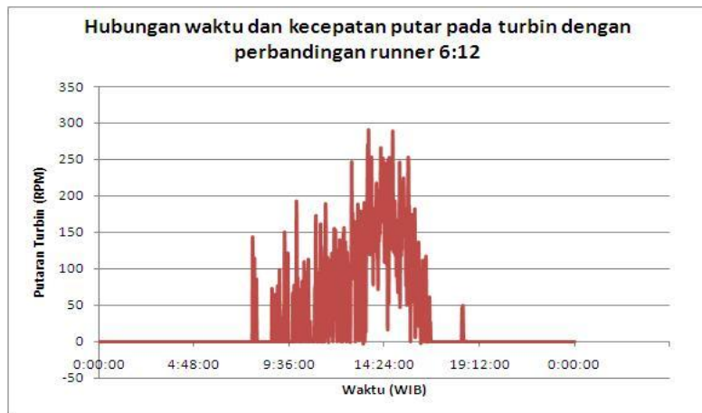
Gambar 5. Hubungan waktu dan kecepatan putar pada rasio jumlah runner 6 : 12
