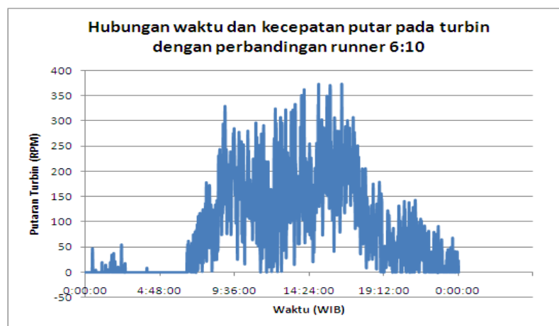
Gambar 4. Hubungan waktu dan kecepatan putar pada rasio jumlah runner 6 : 10
