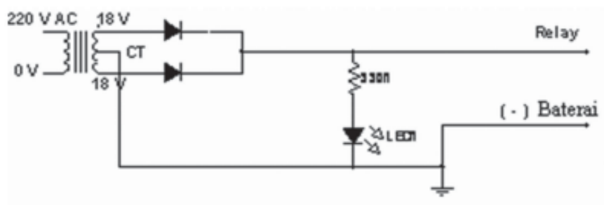
Gambar 4. Rangkaian Pengisian Arus ke Battery
