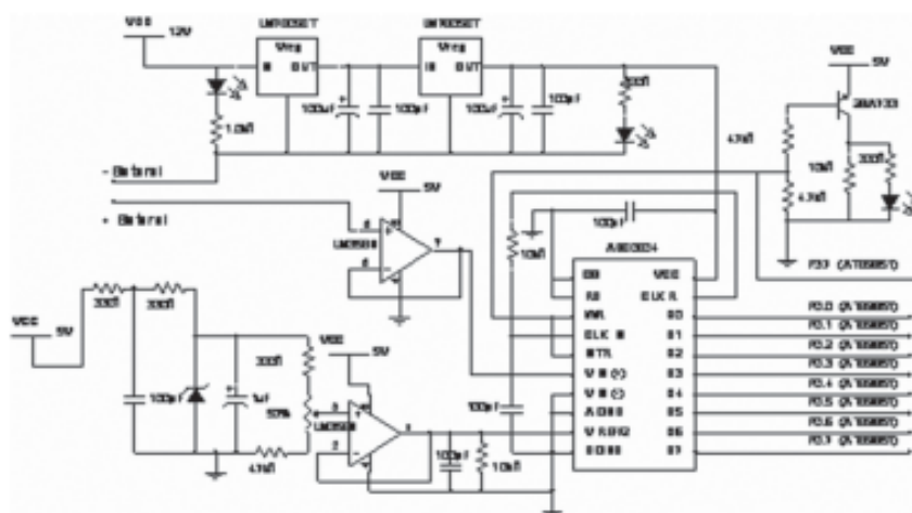
Gambar 8. Rangkaian ADC
