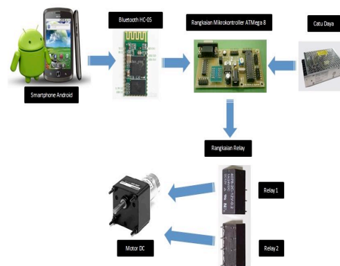
Gambar 2. Diagram Blok Perancangan Perangkat Keras
