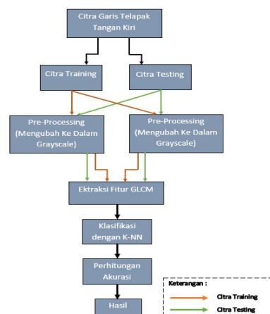
Gambar 5. Skema Proses Pengenalan
