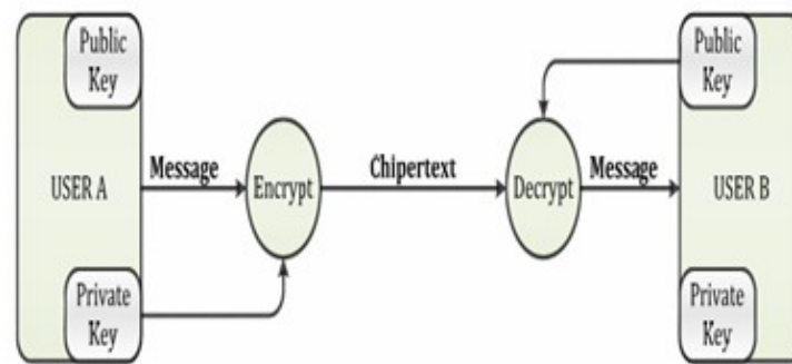
Gambar 5. Proses enkripsi dan dekripsi public-key
