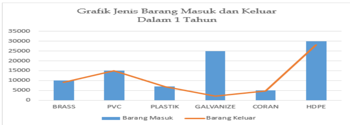
Gambar 6. Diagram HIPO
