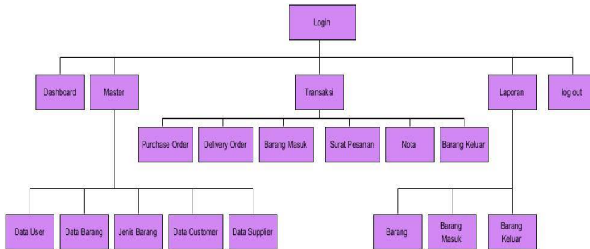
Gambar 7. Diagram HIPO
