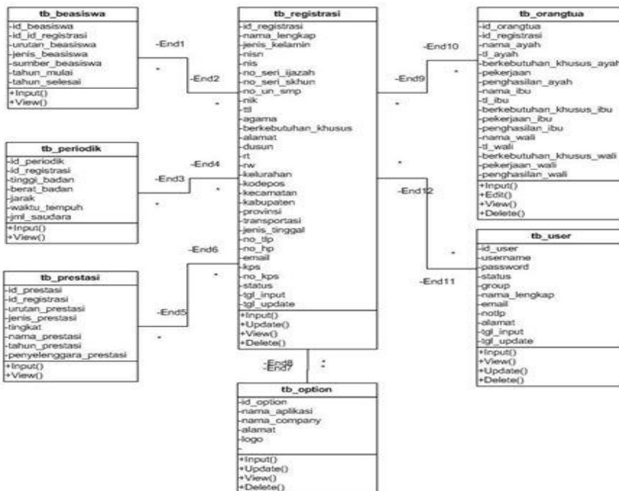
Gambar 4. Class Diagram Pendaftaran Siswa Baru
