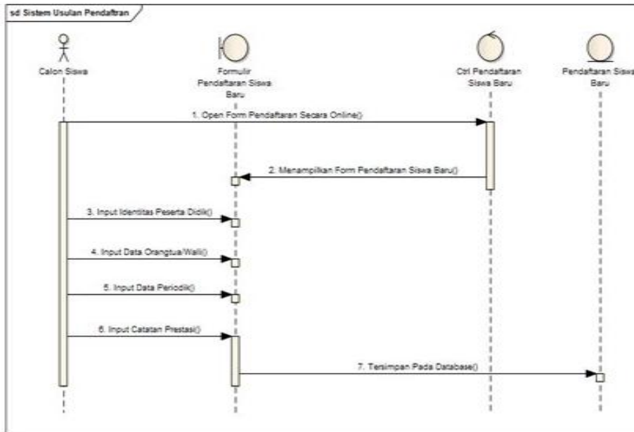
Gambar 3 Sequence Diagram Sistem Usulan Pendaftaran Siswa Baru
