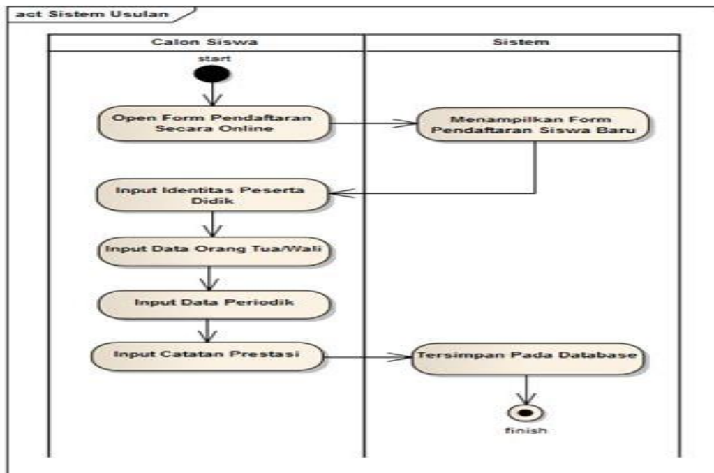
Gambar 2 Activity Diagram Sistem Usulan Pendaftaran Siswa Baru
