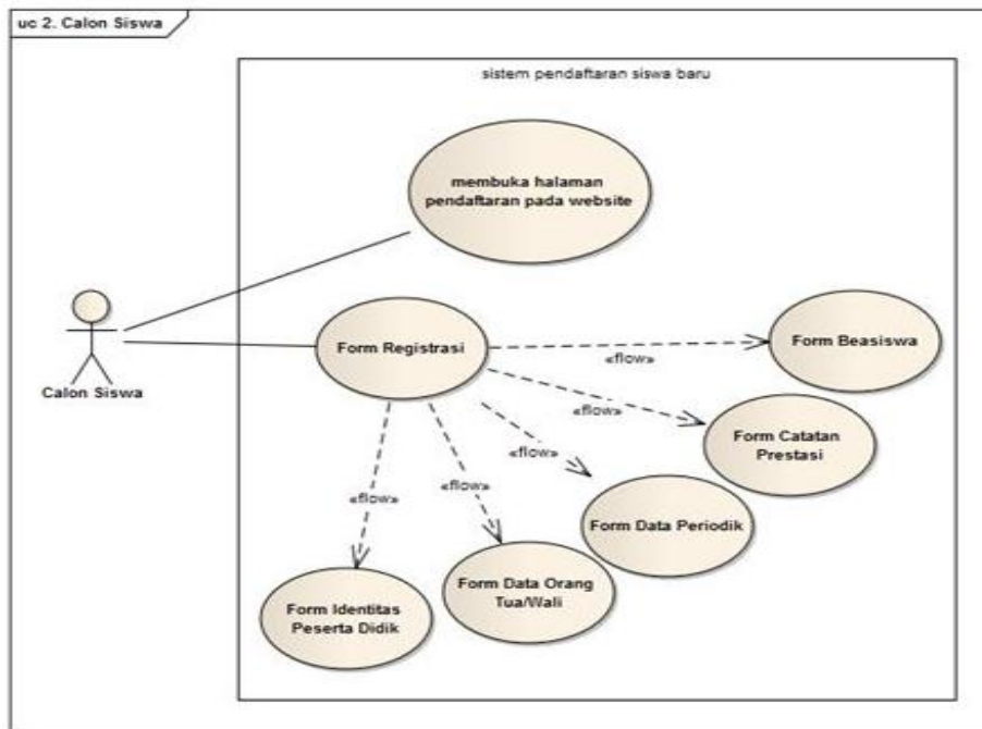
Gambar 1 Use Case Diagram Sistem Usulan Petugas Sekolah
